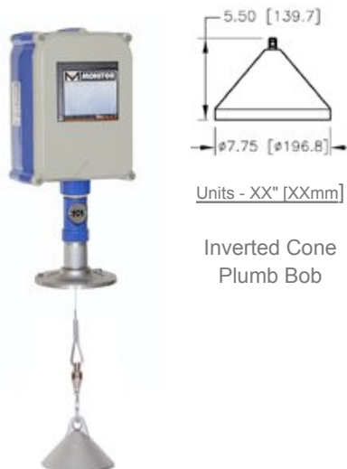
SiloPatrol® SMU
